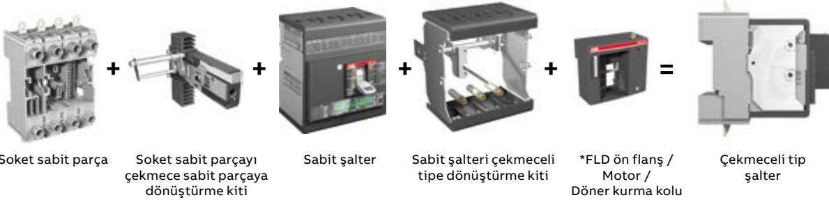
Sabit şalteri çekmeceli tipe dönüştürme kiti
